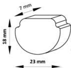
Testata di chiusura a vista anteriore
