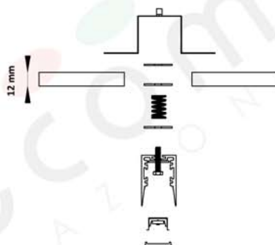
Dettaglio installazione incasso LEVELING SYSTEM
