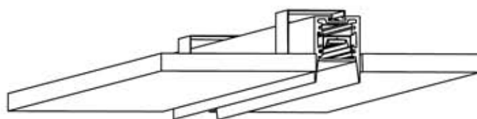
Dettaglio installazione incasso LEVELING SYSTEM
